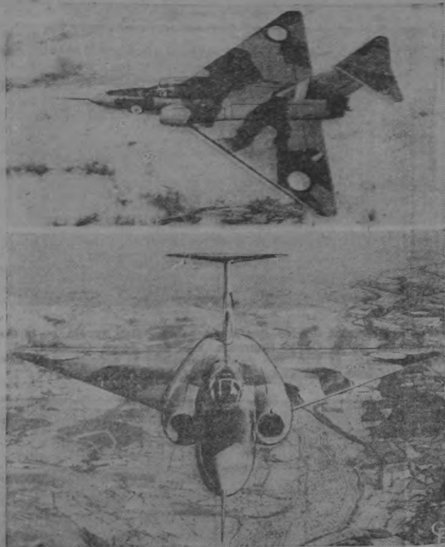
.. El moderno avión británico "Javelin", visto de frente y de lado. Se le considera la máquina "contra la bomba atómica". Está impulsado por dos motores a chorro, cada uno de los cuales produce 8,500 libras de impulso, lo que es equivalente a quince mil caballos de fuerza, en 600 millas por hora, a veinte mil pies de altura.
